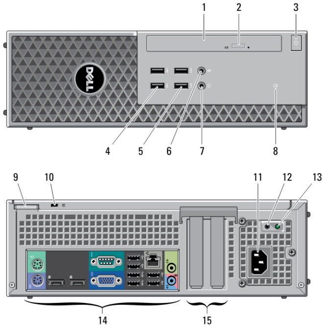
Figur 3. Lite formfaktor sett forfra og bakfra
